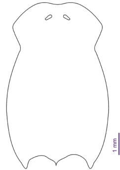
Fig. 1. Vista dorsal de Convolutriloba retrogemma .
