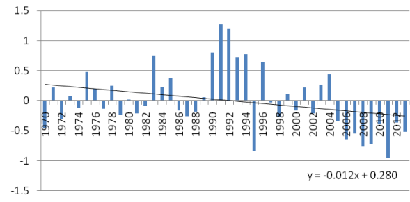
Zona 3 Anomalías de la presión al nivel medio del mar. Agosto 1970-2013
