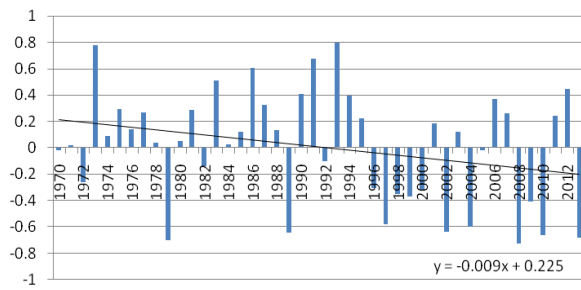
Zona 3 Anomalías de la presión al nivel medio del mar. Septiembre 1970-2013
