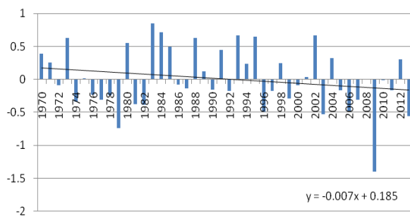
Zona 3 Anomalías de la presión al nivel medio del mar. Noviembre 1970-2013
