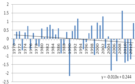
Zona 3 Anomalías de la componente zonal del viento en superficie. Octubre 1970-2013
