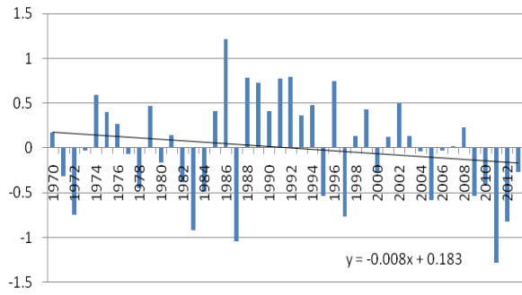
Zona 3 Anomalías de la presión al nivel medio del mar. Julio 1970-2013
