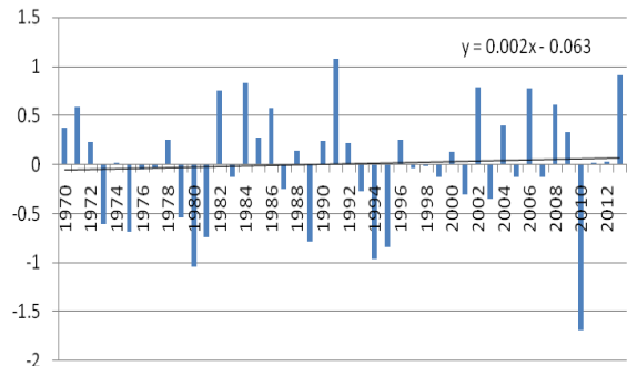
Zona 3 Anomalías de la componente zonal del viento en superficie. Diciembre 1970-2013
