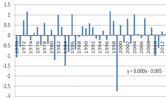
Zona 3 Anomalías de la componente zonal del viento en superficie. Noviembre 1970-2013
