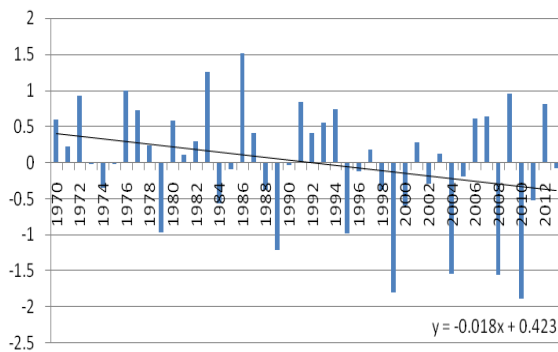
Zona 3 Anomalías de la componente zonal del viento en superficie. Septiembre 1970-2013
