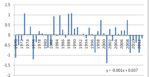
Zona 3 Anomalías de la presión al nivel medio del mar. Diciembre 1970-2013
