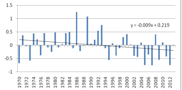
Zona 3 Anomalías de la presión al nivel medio del mar. Octubre 1970-2013
