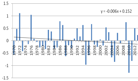
Zona 3 Anomalías de la componente zonal del viento en superficie. Julio 1970-2013
