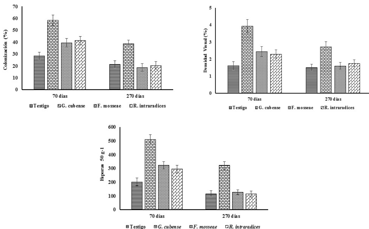
Las barras verticales muestran el intervalo de confianza de la media. Intervalos de confianza que se solapan entre si no difieren significativamente ( \alpha = 0,05 ). Cepas de HMA: Glomus cubense , Funneliformis mosseae , Rhizophagus intraradices
