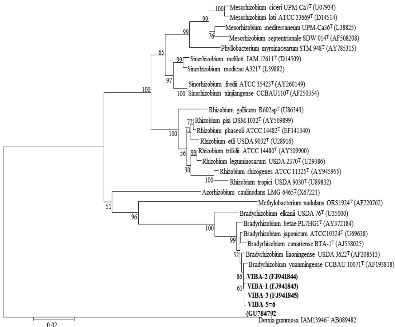
Figura 3. Árbol filogenético derivado de la alineación de 1484 pb del gen 16S rDNA de los tipos de cepas aislados y los más representativos
