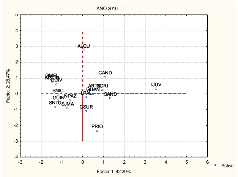
Figura 11. Distribución de los individuos según las componentes principales, período 5, Año 2010
