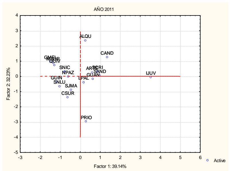
Figura 12. Distribución de los individuos según las componentes principales, período 5, Año 2011
