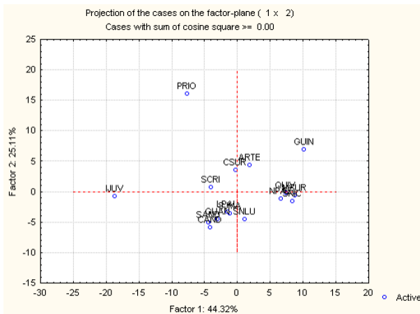
Figura 4. Representación de los individuos en las dos primeras componentes principales del ACPFM.
