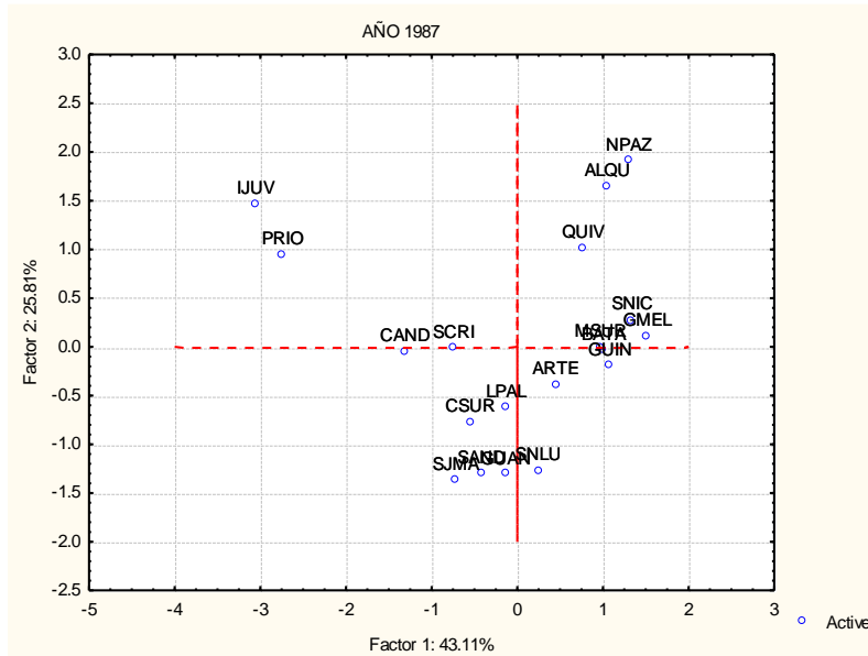
Figura 5. Distribución de los individuos según las componentes principales, período 1 Período 2 1983 – 1990
