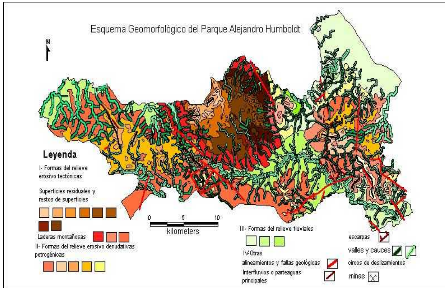
Fig. II.3 Esquema geomorfológico.
