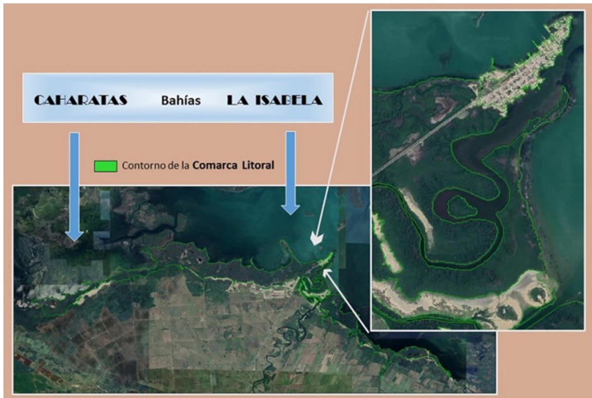
Figura 11 Ventana de la comarca litoral Caharatas-Playa Uvero en el municipio Sagua la Grande, con fachada en la costa en el centro norte de Cuba. Véase la conurbación del poblado La Isabela, que en dependencia de la escala de trabajo será distinguida del resto de las «Tierras Litorales». Según Hernandez et al. , 2021
