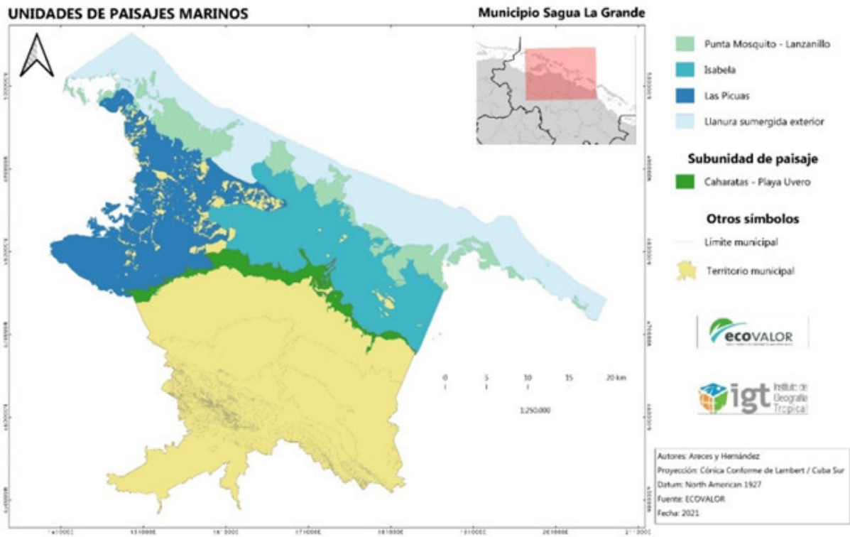
Figura 9 Paisajes marinos y la comarca litoral, una subunidad de paisaje terrestre íntimamente asociada al borde costero, en un polígono de trabajo del litoral centro norte de Cuba. En condiciones de naturalidad muy elevada, la comarca litoral puede coincidir con las Tierras Litorales. Según Hernandez et al.,2021
